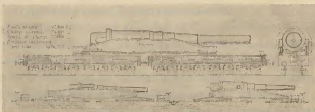
Fig. 16 — Vagões especiais para o transporte de canhões
