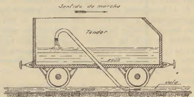
Fig. 13 — Croquis explicativo da toma de água em trânsito
