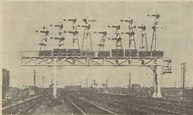
Fig. 20 — Ponte de sinais para vias divergentes
