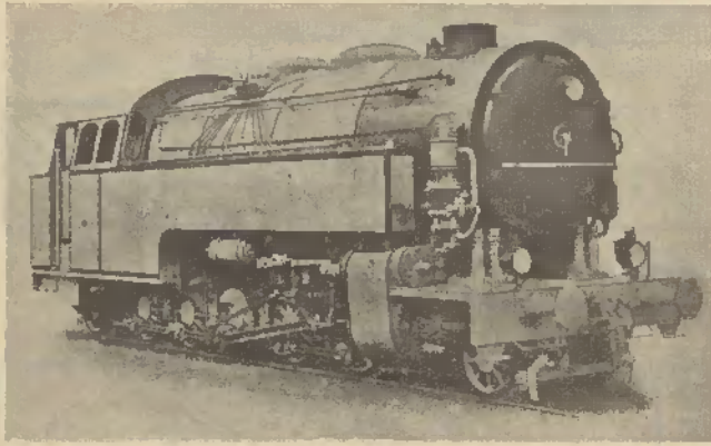
Fig. 11 — Locomotiva-tender alemã
